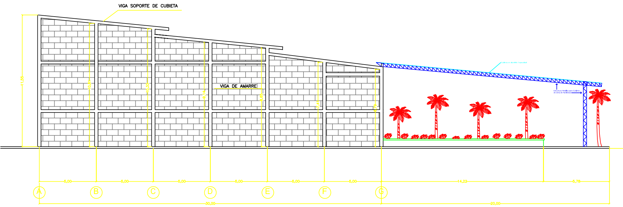
FACHADA LATERAL BODEGA
